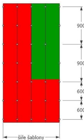
Rohová oblast po 600 mm do každé vlny
