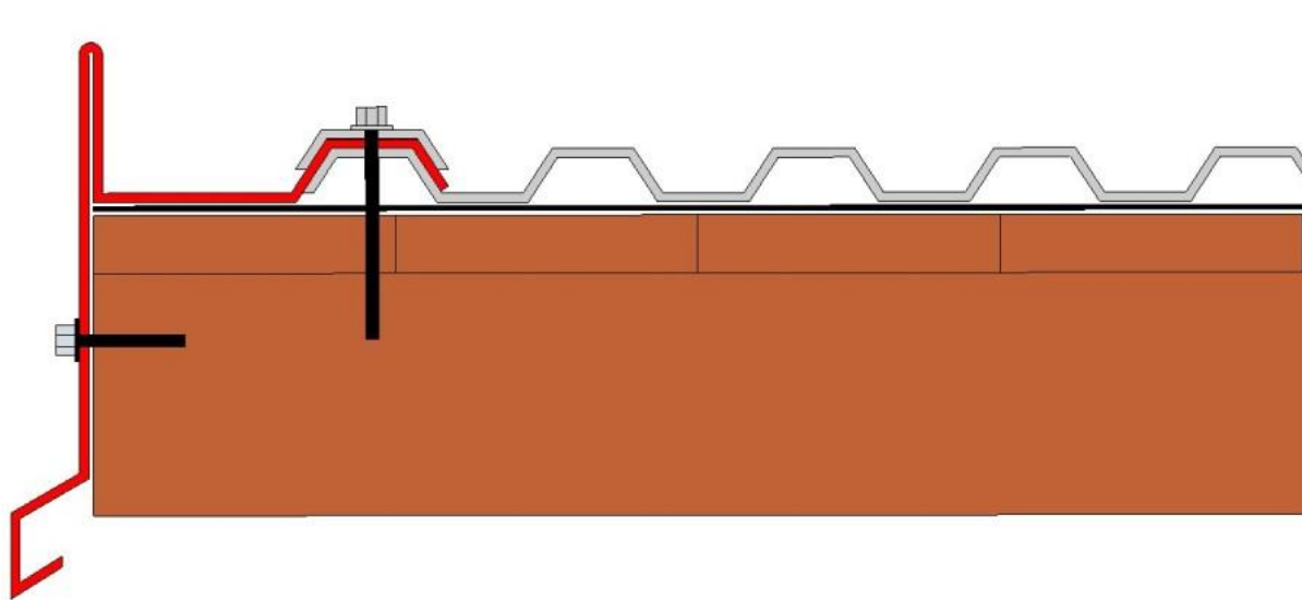
Výkres 8a: Závětrná lišta
