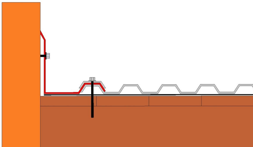
Výkres 6a: Boční lišta
