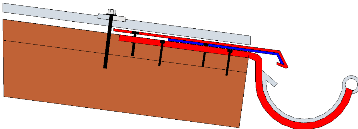
Výkres 1a: Detail odkapní hrany
