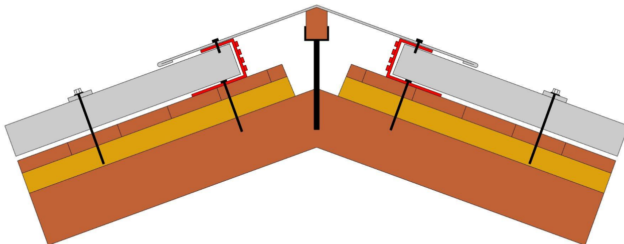
Výkres 4: Detail větraného hřebenáče
