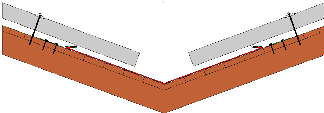
Výkres 5: Detail úžlabí
