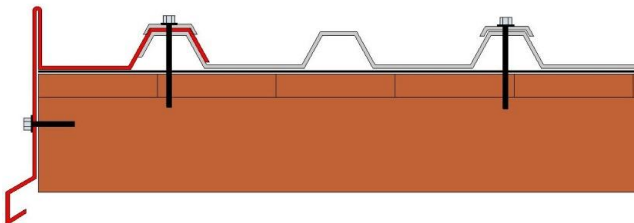
Výkres 10b: Závětrná lišta
