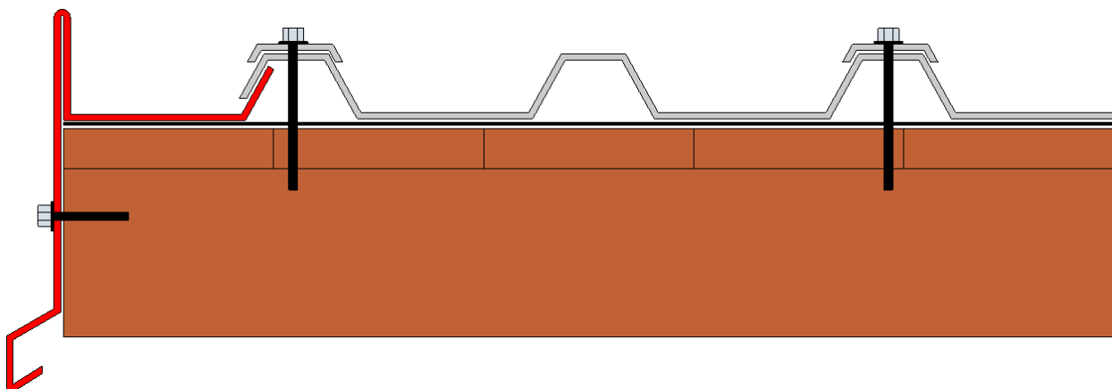
Výkres 9a: Závětrná lišta
