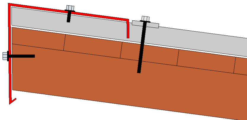
Výkres 6: Závětrná lišta čelní k pultové střeše
