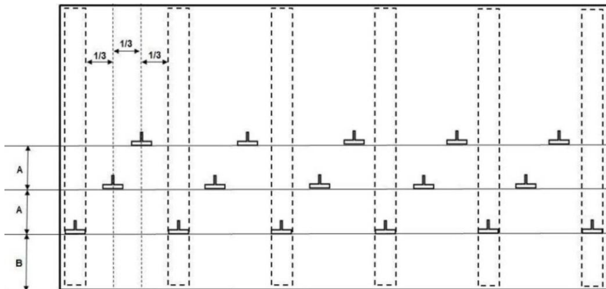
Výkres 12: Rozmístění sněhových zábran
