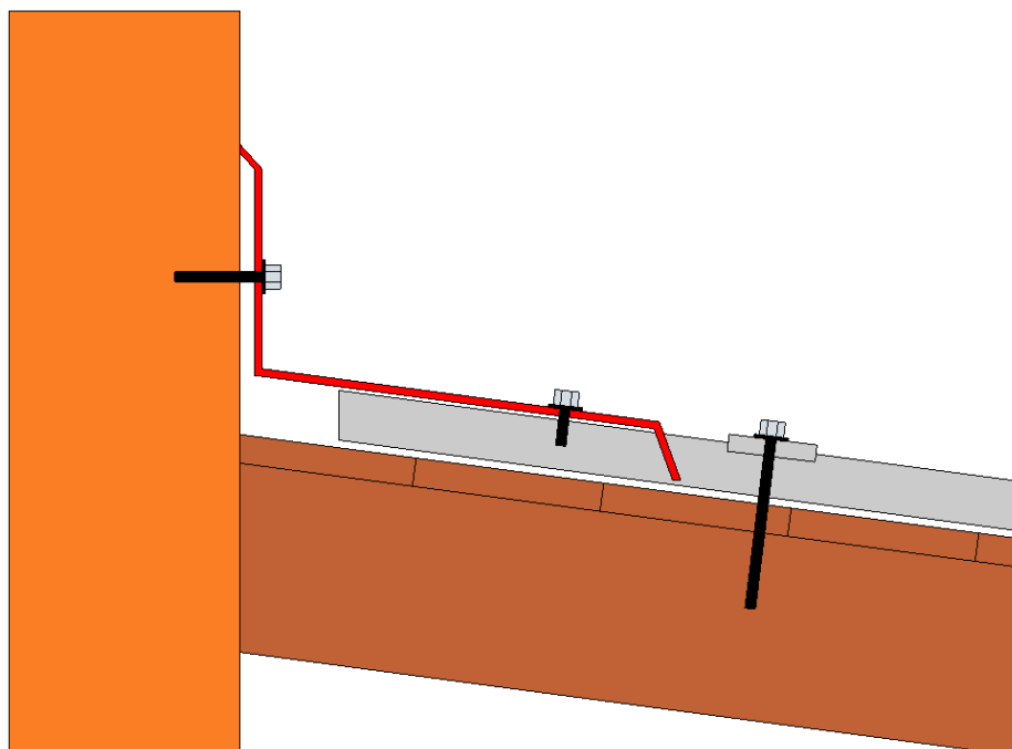
Výkres 11: Lišta ke zdi čelní - horní
