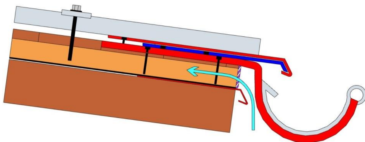
Výkres 2b: Detail odkapní hrany s větranou mezerou
