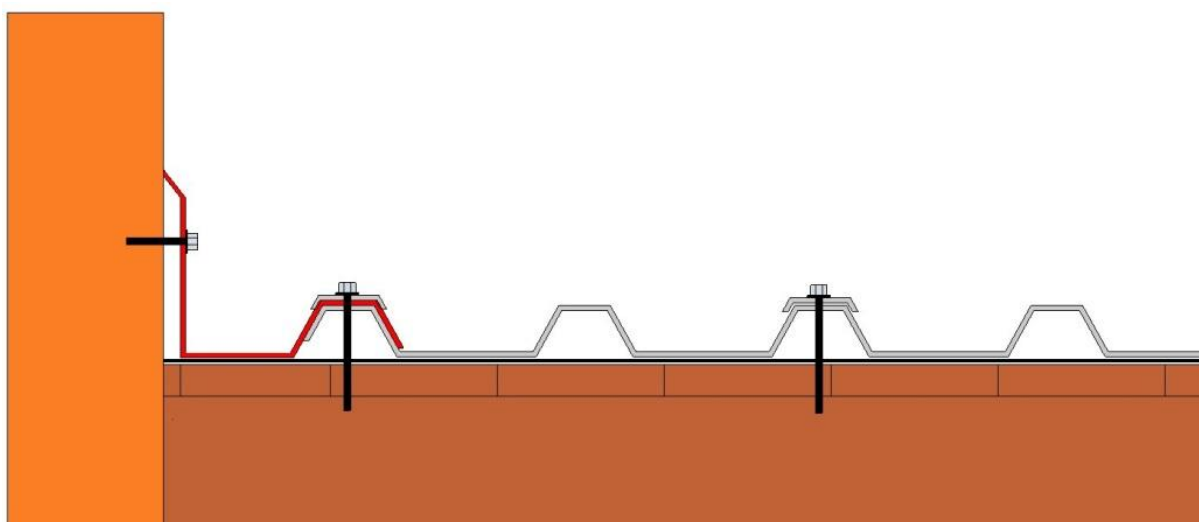
Výkres 8b: Boční lišta
